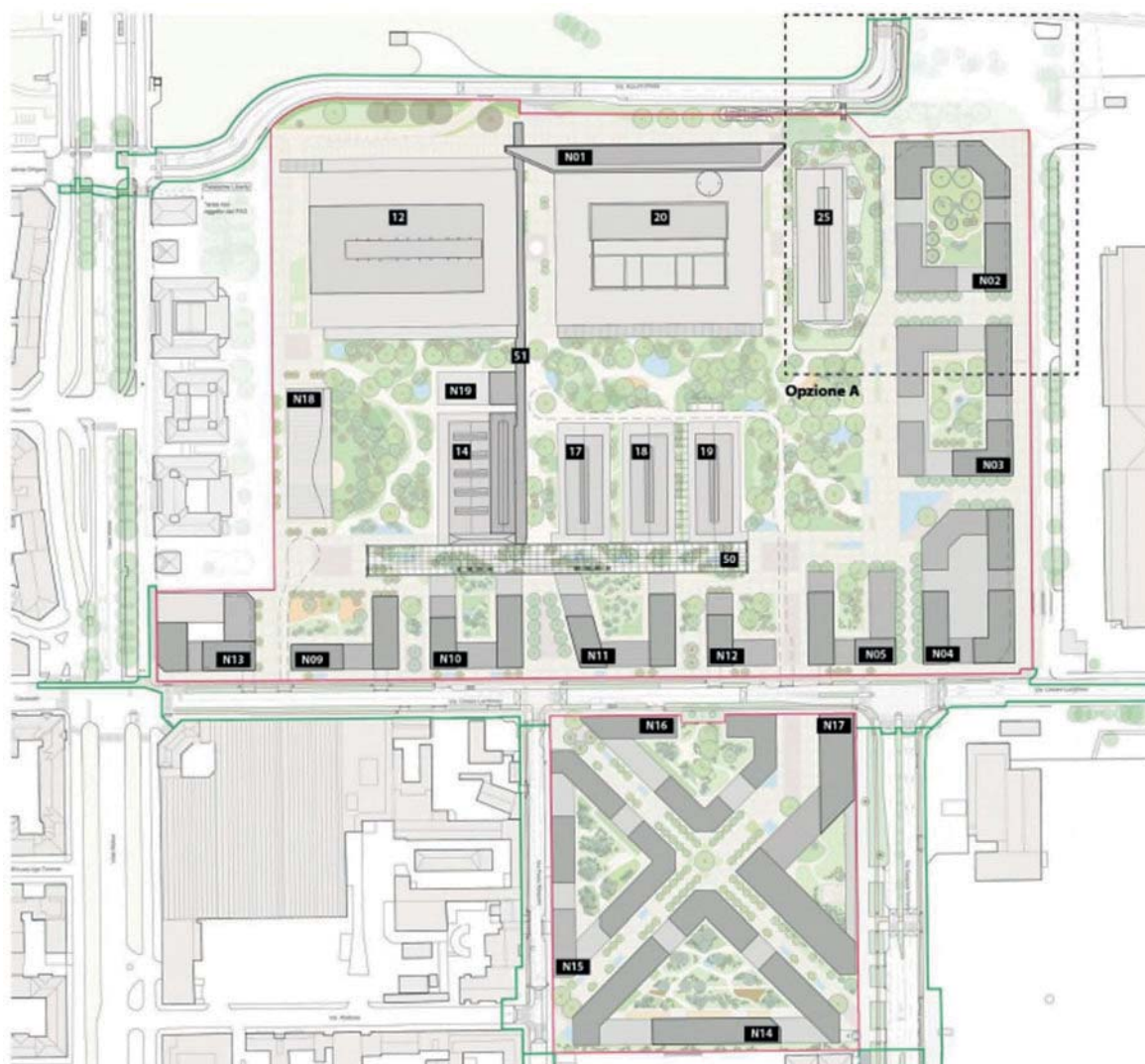
Figura 2—8. Planimetria generale
